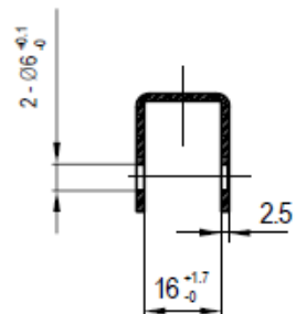
Saddle 1:1
